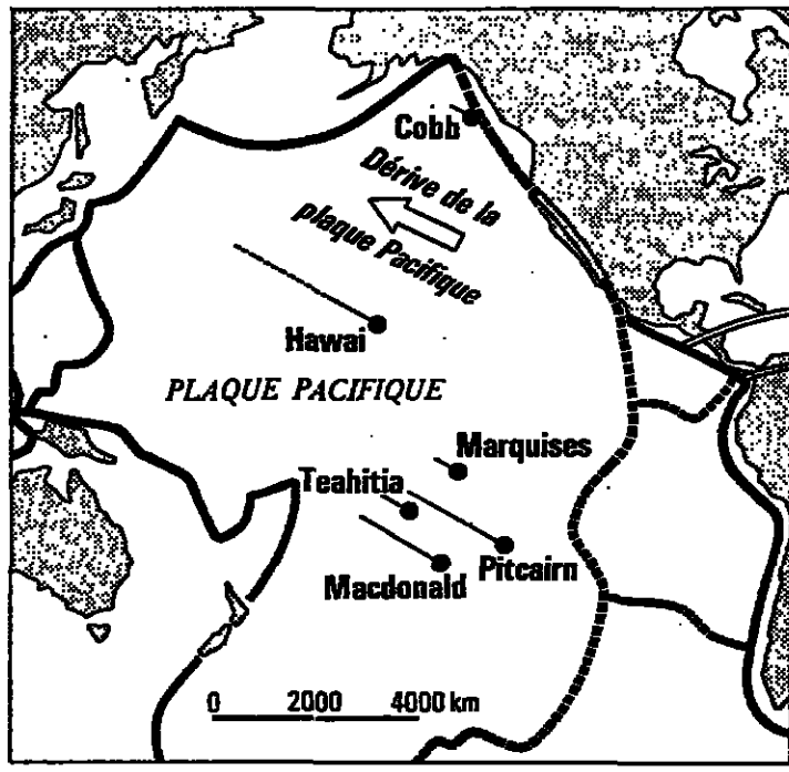
● Point chaud — Fossé océanique — Alignement de volcans — Dorsale océanique — Faille transformante (mouvement latéral)
